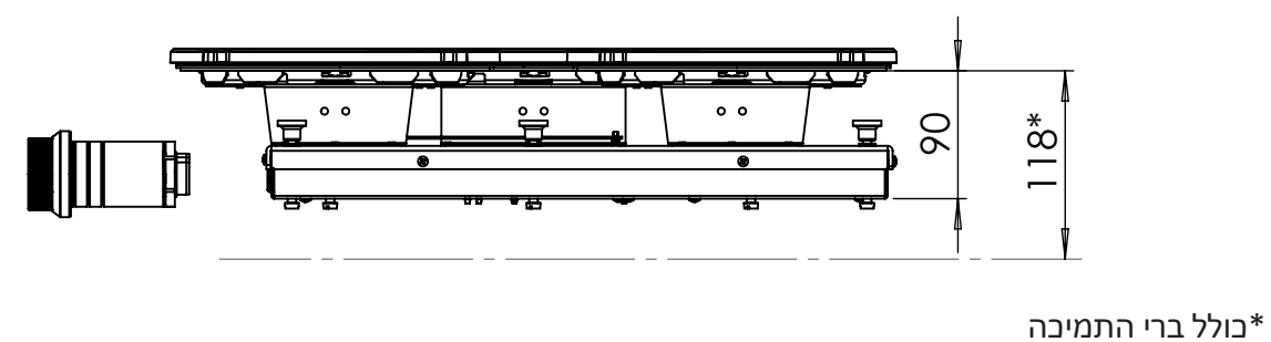
מבט צדדי
