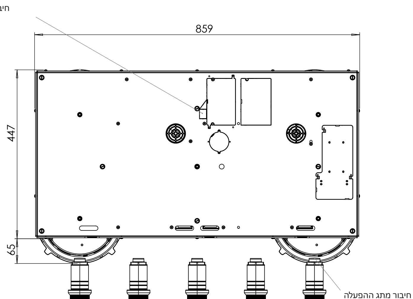
מבט תחתון
