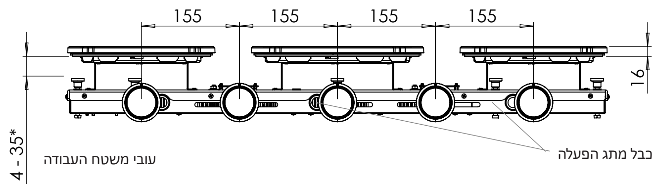
מבט חזיתי
